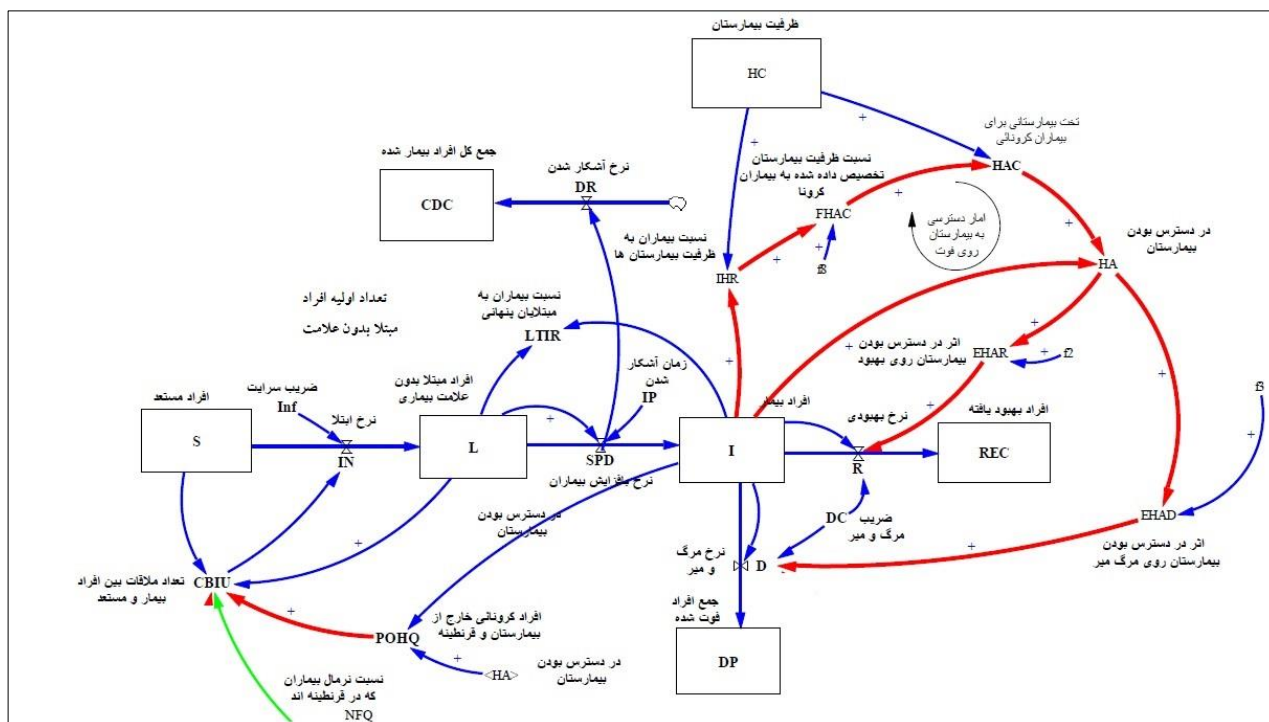
شکل ۱: الگوی کروناونسیم
